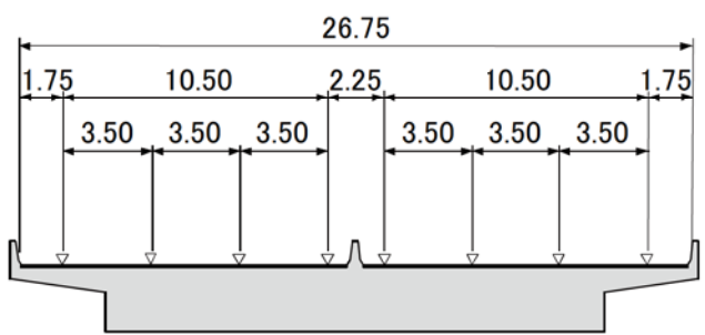
大阪湾岸道路西伸部 標準横断面図 (単位 : m)
