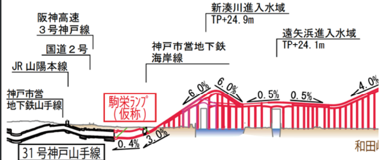
大阪湾岸道路西伸部 縦断面図 (※構造については、現時点の計画であり、今後)
